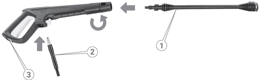
Рисунок 2. Схема встановлення розпилювального тракту високого тиску.
