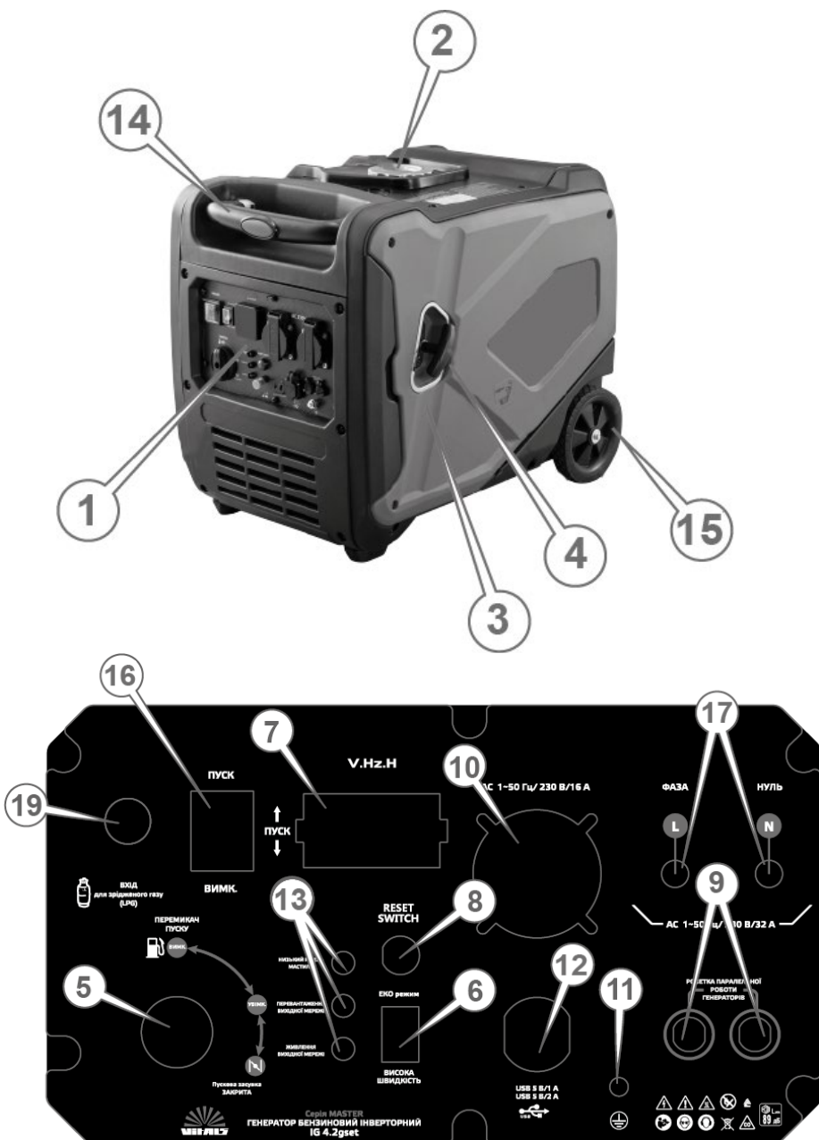
Рисунок 1. Загальний вигляд виробу та панелі керування.
